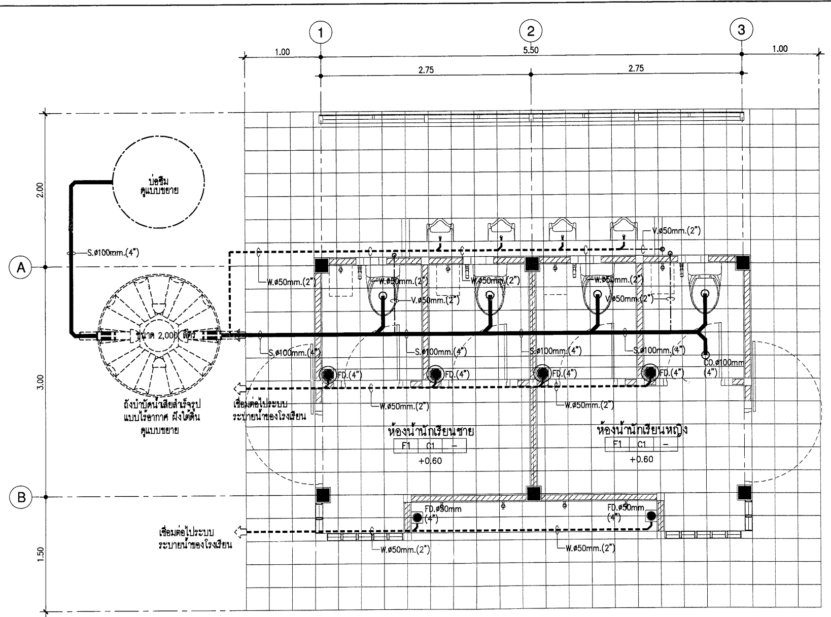
แปลนน้ำเสีย
