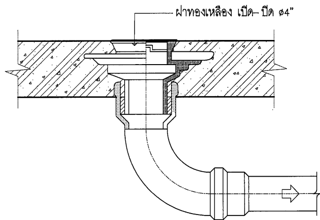
แบบขยาย CO. ไม่กำหนดมาตราส่วน
